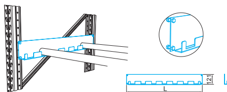
21 Кронштейн для труб ø 50 мм
