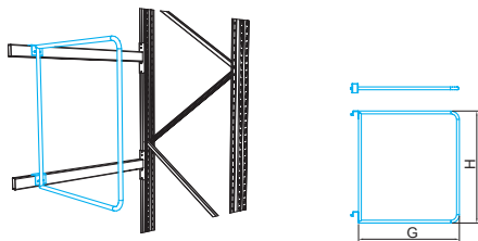
18 Разделитель рамный Н-1000
