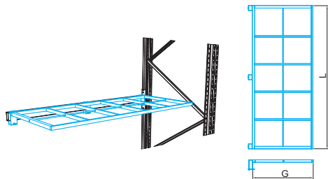
17 Разделитель из сетки
