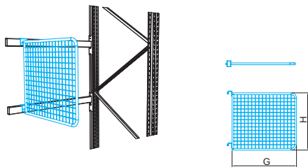
19 Разделитель рамный из сетки Н-800
